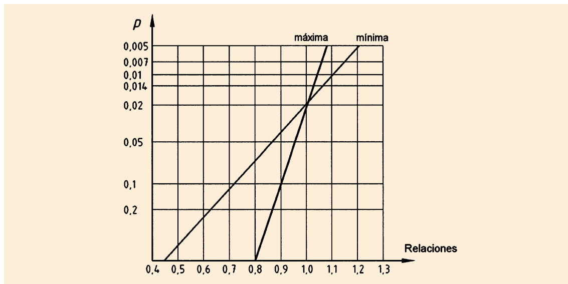
FIGURA 4.3-c RELACIONES T_{max,p} / T_{max} Y T_{min,p} / T_{min}
