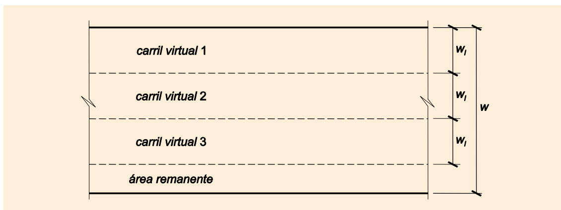
FIGURA 4.1-a EJEMPLO GENÉRICO DE DISTRIBUCIÓN DE CARRILES VIRTUALES
