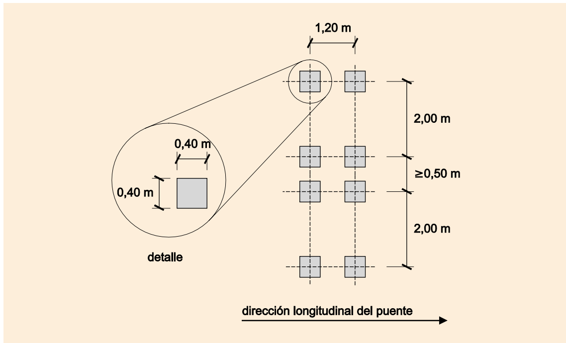
FIGURA 4.1-c DISPOSICIÓN DE VEHÍCULOS PESADOS PARA COMPROBACIONES LOCALES
